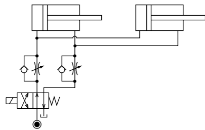
【Meter-in Circuit】
