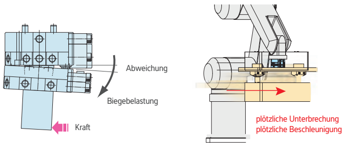
BELASTUNGSTEST UNTER EINEM BIEGEMOMENT (bei Druckluft 5bar)
