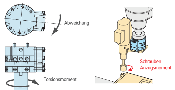
BELASTUNGSTEST UNTER EINEM TORISIONSMOMENT (bei Druckluft 5bar)
