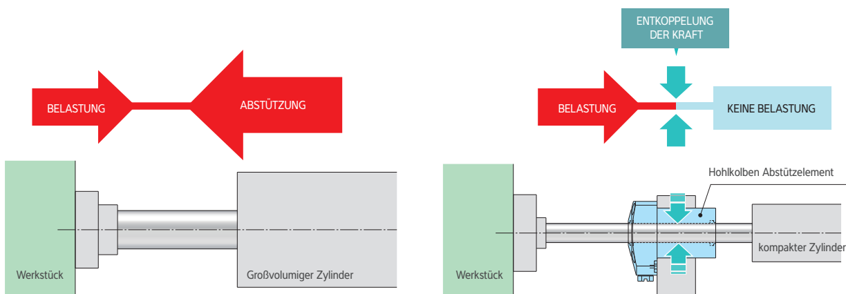
Hohlkolben Abstützelement
